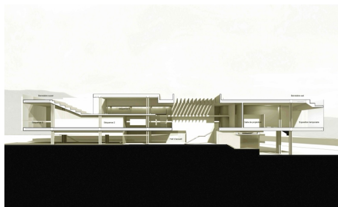
Coupe perspective de principe du musée de Mariana, 2012. © Agence Faloci
